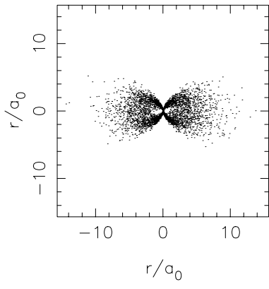
\psi_{311}
