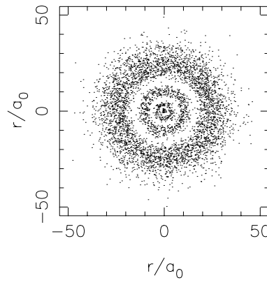
\psi_{400}
