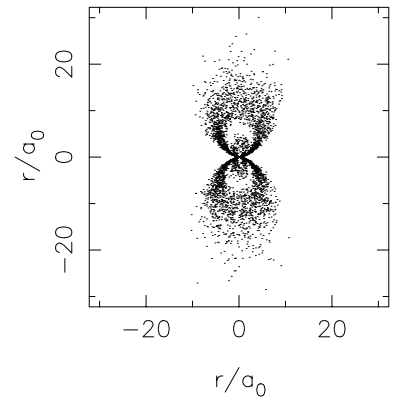
\psi_{321}
